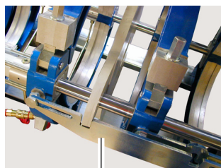
Mechanizm zwalniający
